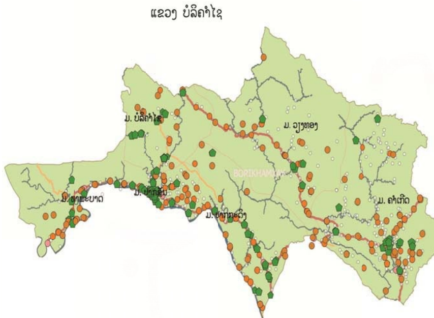
ຮູບສະແດງ 32: ເຄືອຂ່າຍຮັບ-ສົ່ງສັນຍານໂທລະສັບມືຖືຂອງບັນດາບໍລິສັດ, ແຂວງ ບໍລິຄຳໄຊ
